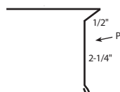
22b 4" DRIP EDGE
